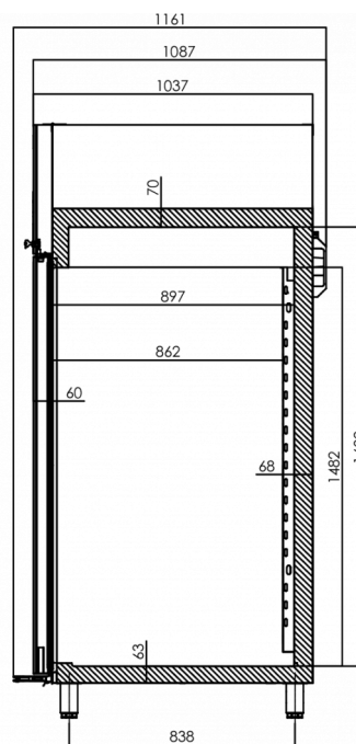
SECTION A-A
