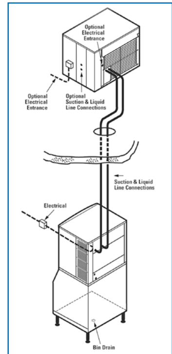
Beispielhafte QuietTube-Installation
