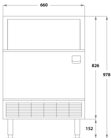
Frontansicht
