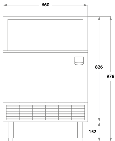
Frontansicht
