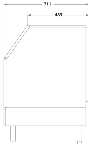
Seitenansicht
