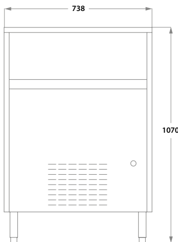
Frontansicht
