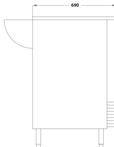
Seitenansicht
